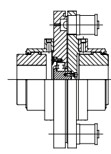
FET/FSUET ESCO TORQUE C4230a Page 47
